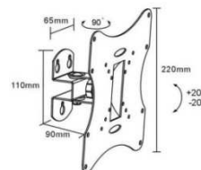
1 support pré-assemblé
